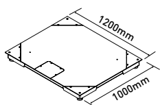
Xtrem Lion-S 1210
