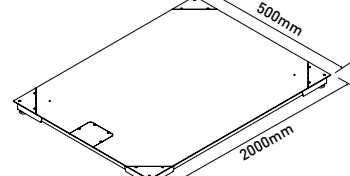
Xtrem Lion-S 2015
